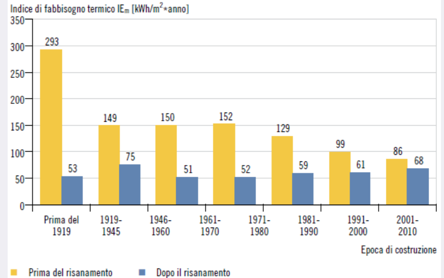
Confronto tra indici di fabbisogno di energia termica IE_m prima e dopo un risanamento energetico
