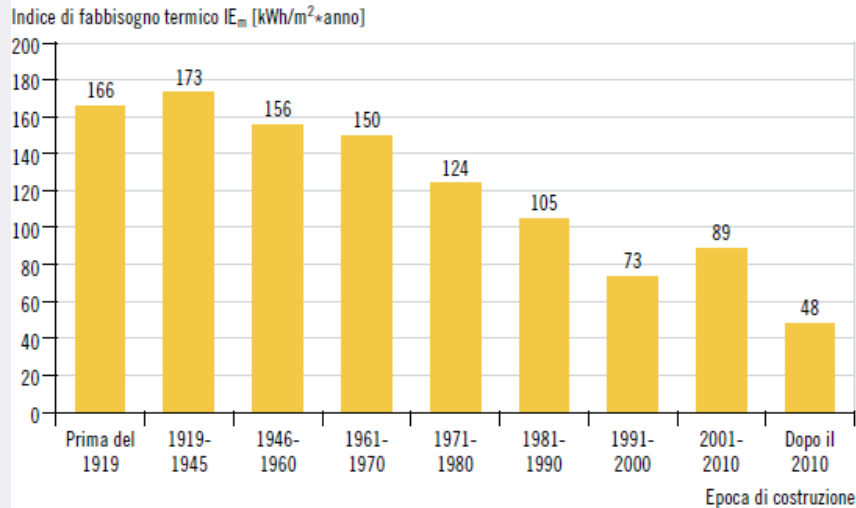
Indice di fabbisogno annuo di energia termica IE_m per gli edifici residenziali in Cantone Ticino
