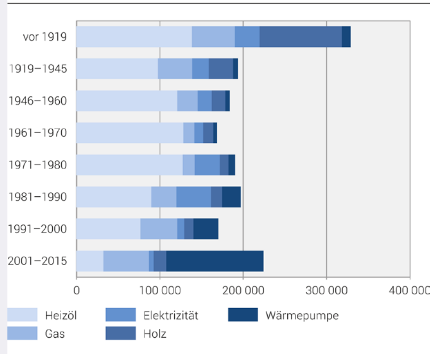
Die wichtigsten Energieträger der Heizung nach Alter der Gebäude, 2015
